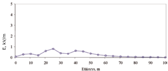
Kuva 5. Sähkökentän mittaustuloksia sähköaseman ulkopuolelta aseman aidasta lähtien.
